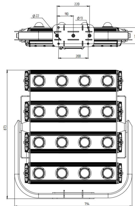
Рисунок 2. Габаритный чертеж
